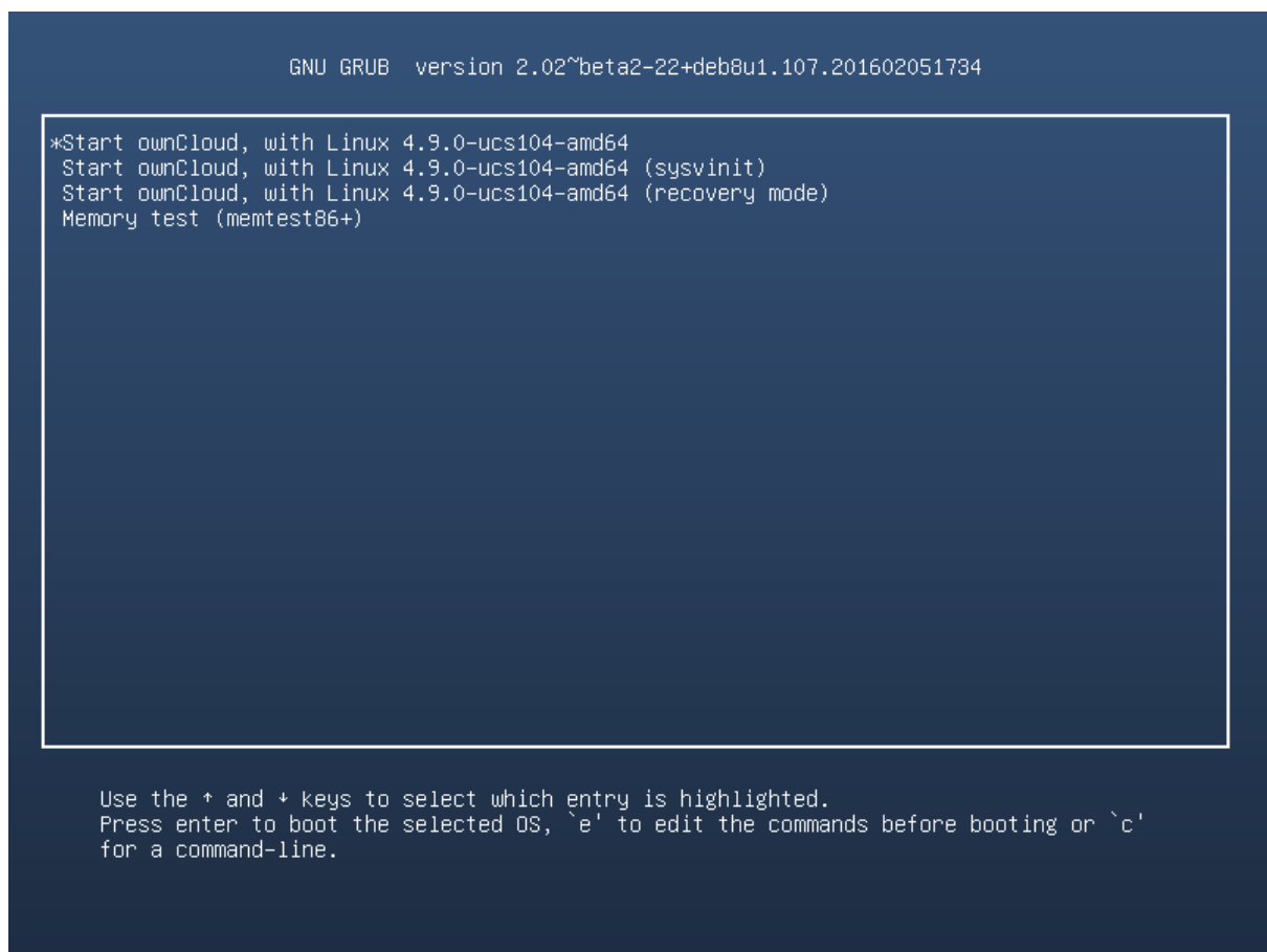
Fig. 7.1: Boot loader
