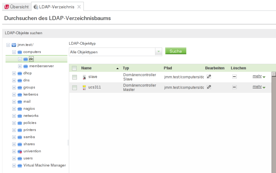
Abbildung 4.5. Navigation im LDAP-Verzeichnis
