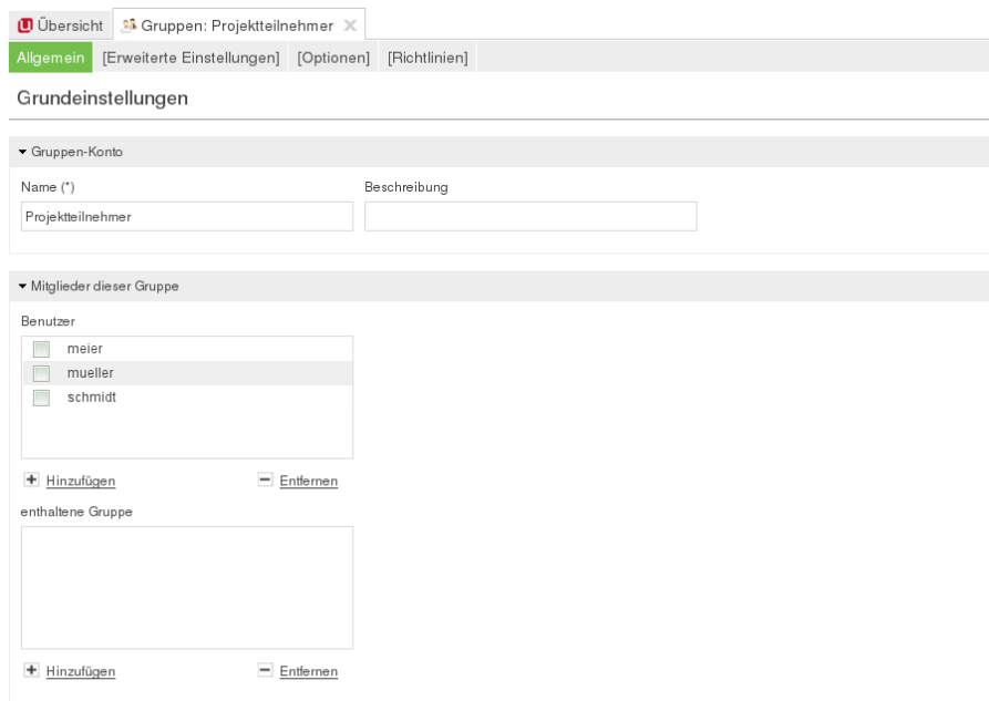
Abbildung 6.1. Anlegen einer Gruppe in UMC
