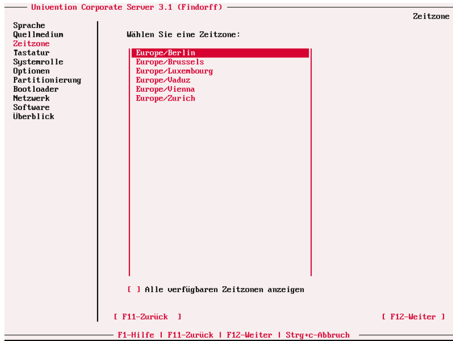
Abbildung 2.3. Auswahl der Zeitzone
