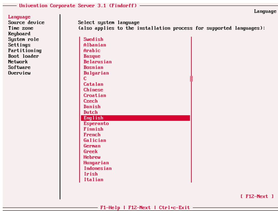
Abbildung 2.2. Auswahl der Installationsssprache
