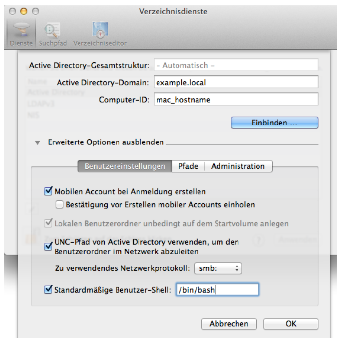
Abbildung 3.2. Domänenbeitritt eines Mac OS X-Systems
