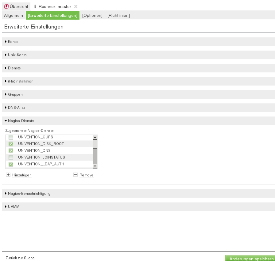
Abbildung 13.3. Zuweisung von Nagios-Prüfungen zu einem Rechner
