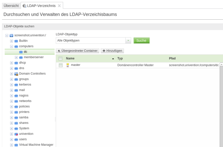
Abbildung 4.5. Navigation im LDAP-Verzeichnis
