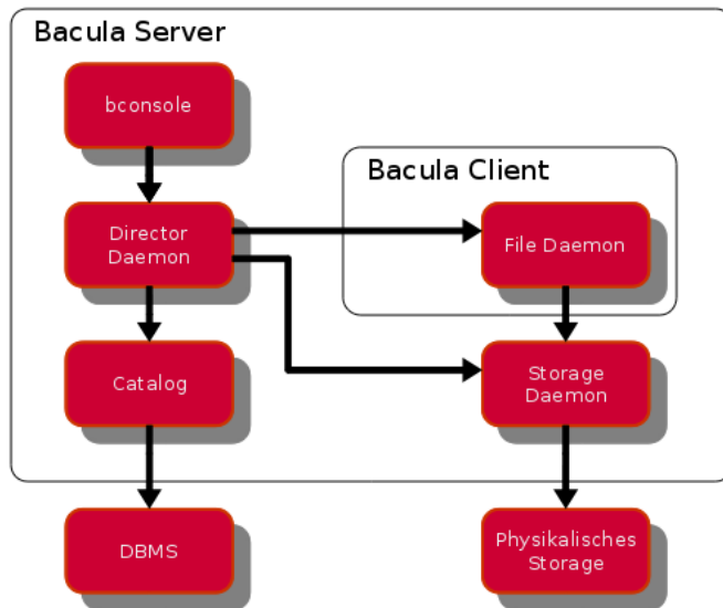
Abbildung 16.1. Bacula Schema
