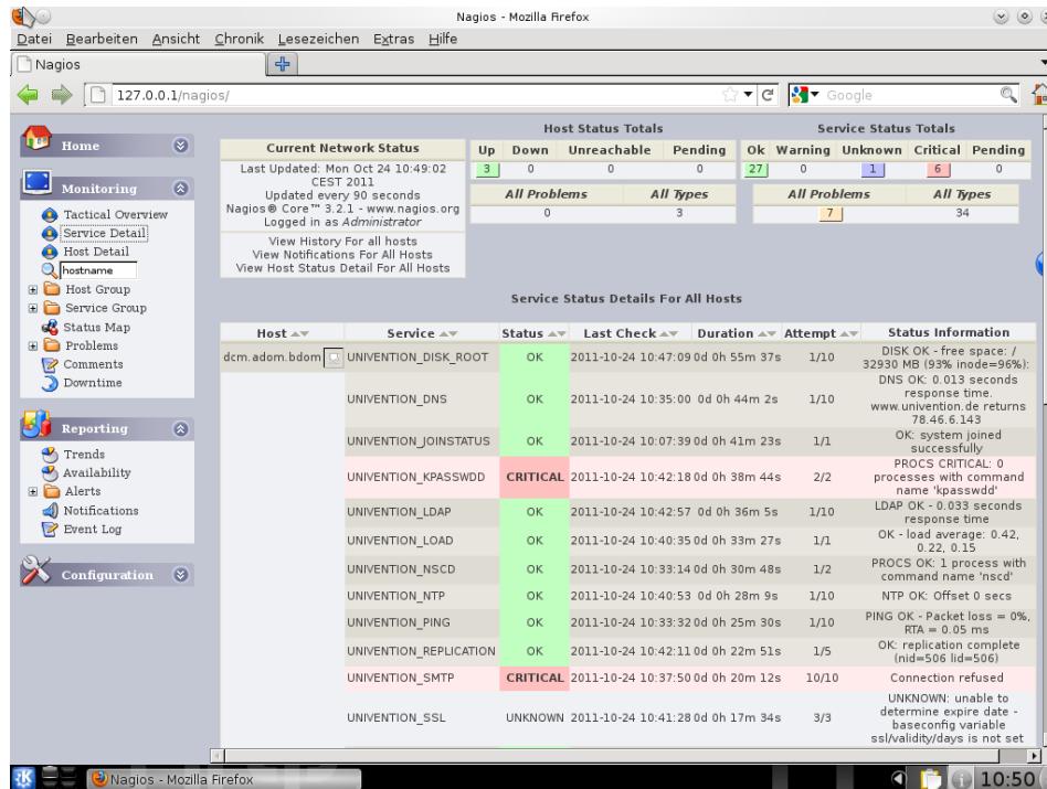
Abbildung 14.1. Nagios Status-Webinterface
