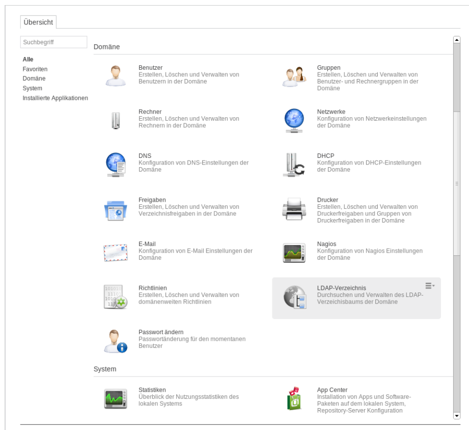
Abbildung 4.3. Modulübersicht
