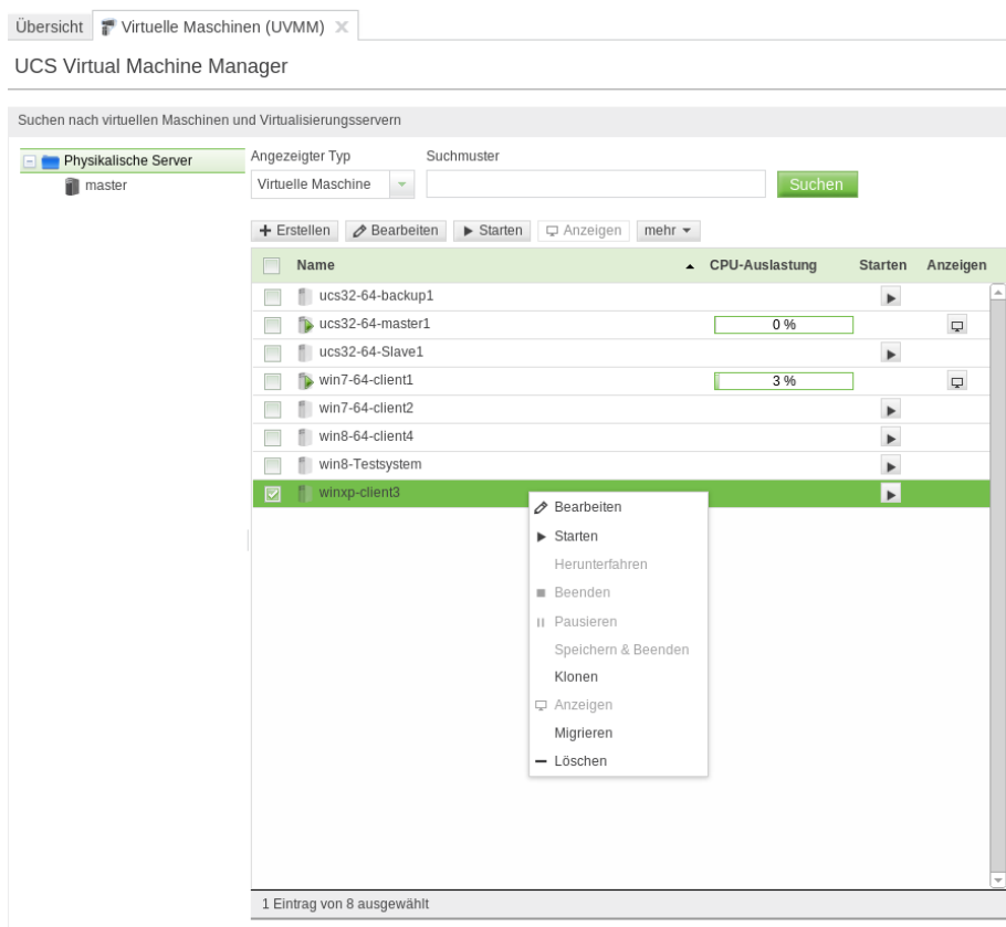
Abbildung 15.3. Übersicht über die virtuellen Maschinen
