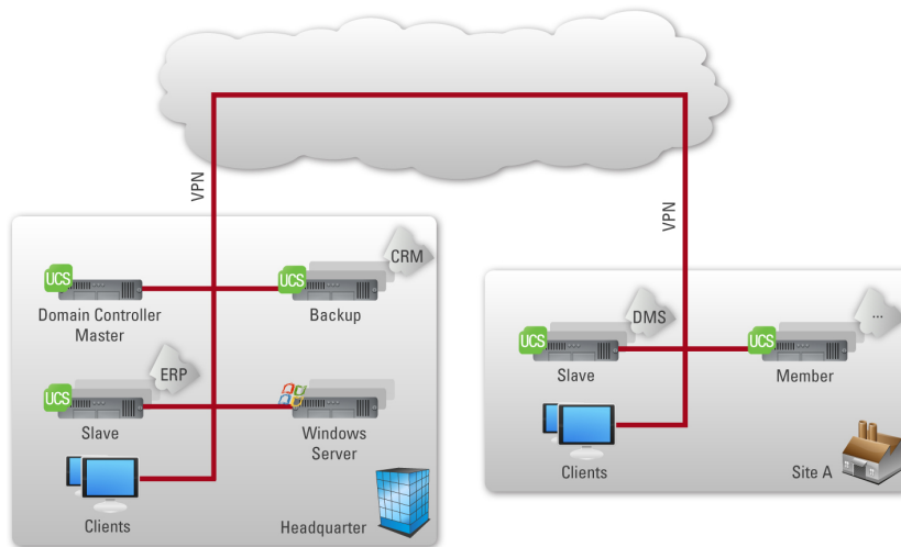
Abbildung 1.1. UCS-Domänenkonzept
