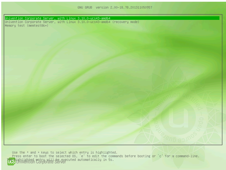
Abbildung 8.1. GRUB-Auswahlmenü
