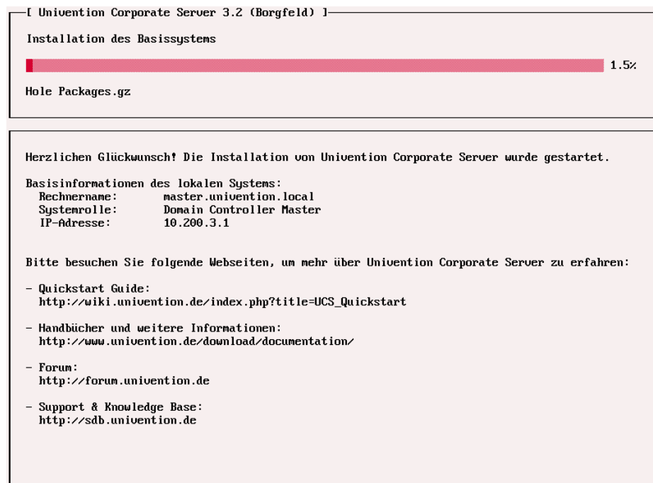
Abbildung 2.11. Installationsfortschritt
