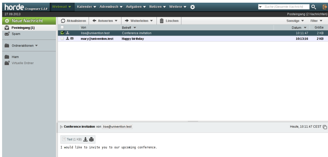
Abbildung 13.5. Webmail (Posteingang)
