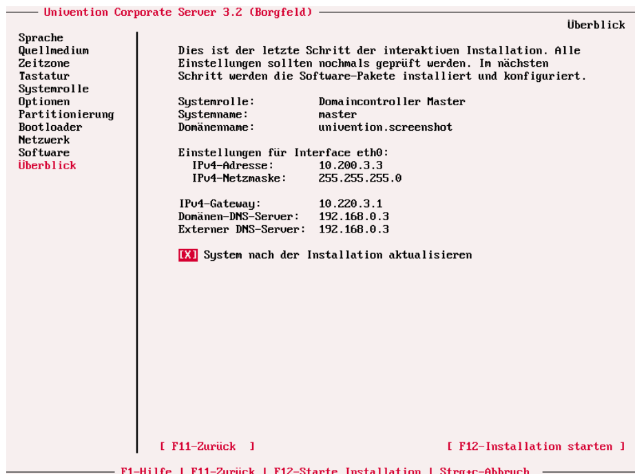
Abbildung 2.10. Installationsüberblick
