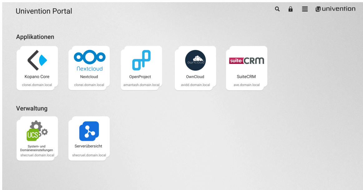
Abbildung 4.1. UCS Portalseite
