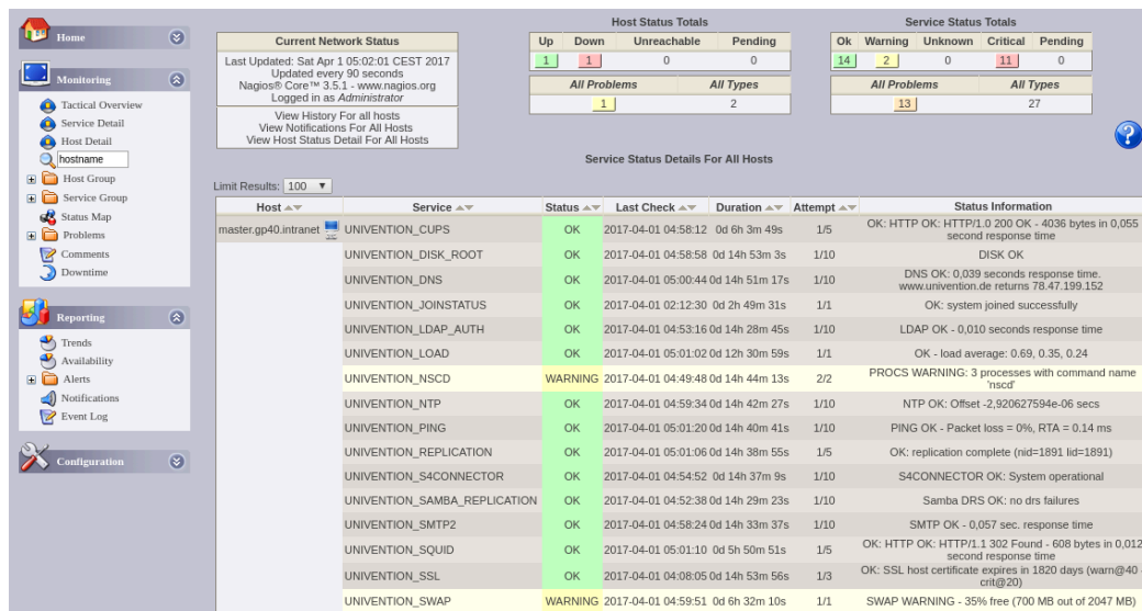
Abbildung 15.1. Nagios Status-Webinterface
