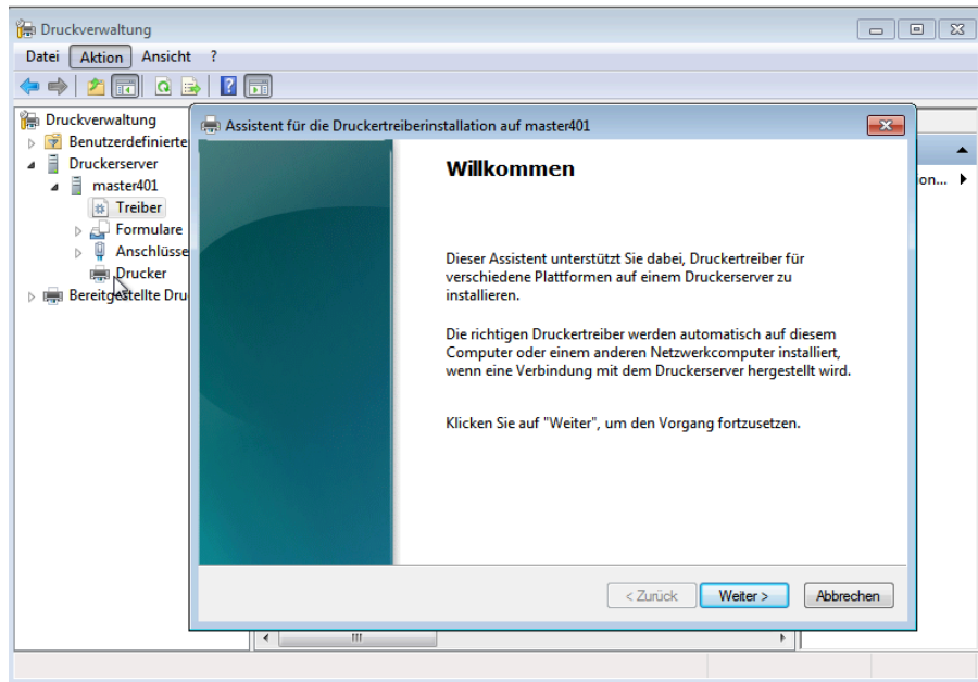
Abbildung 13.6. Treiberinstallation
