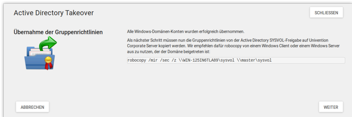
Abbildung 9.12. Kopieren der Sysvol-Freigabe
