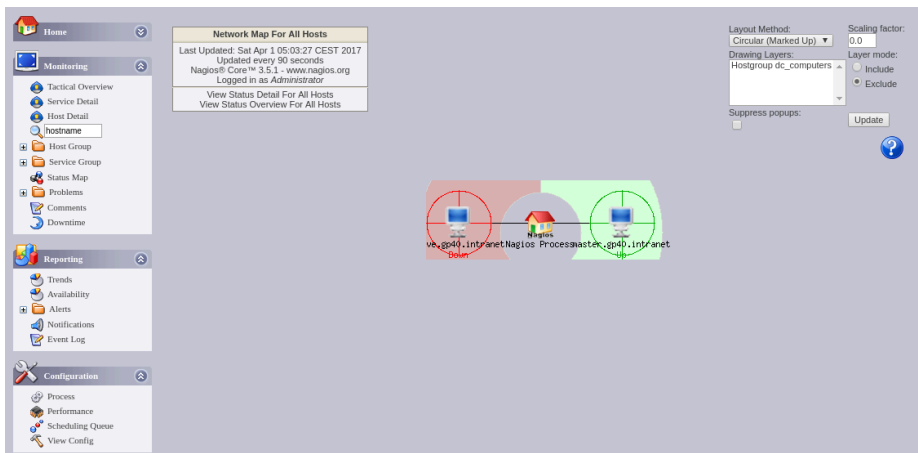
Abbildung 15.4. Nagios-Statusübersicht
