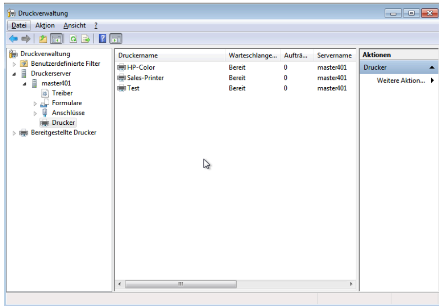
Abbildung 13.5. Druckerliste
