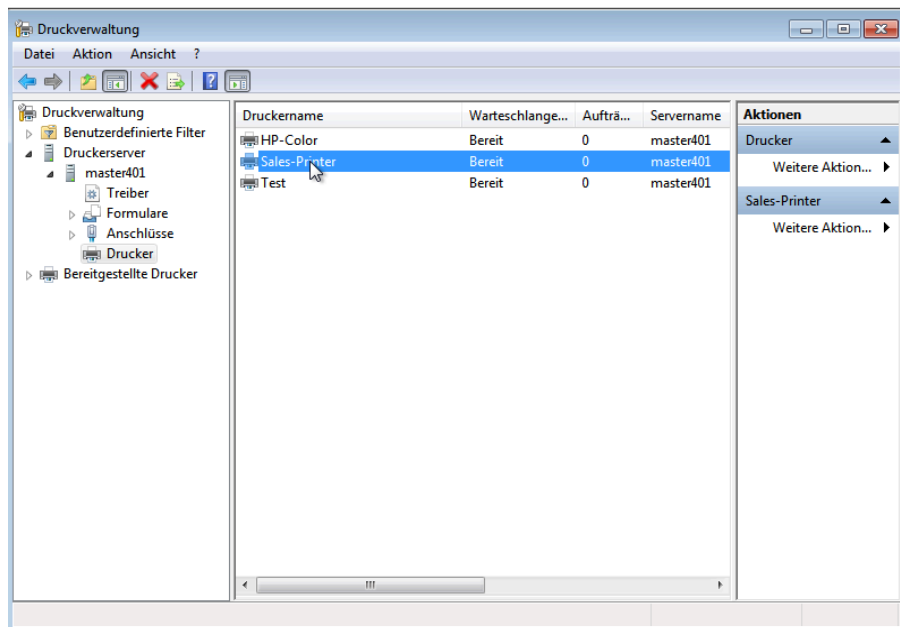
Abbildung 13.7. Drucker auswählen
