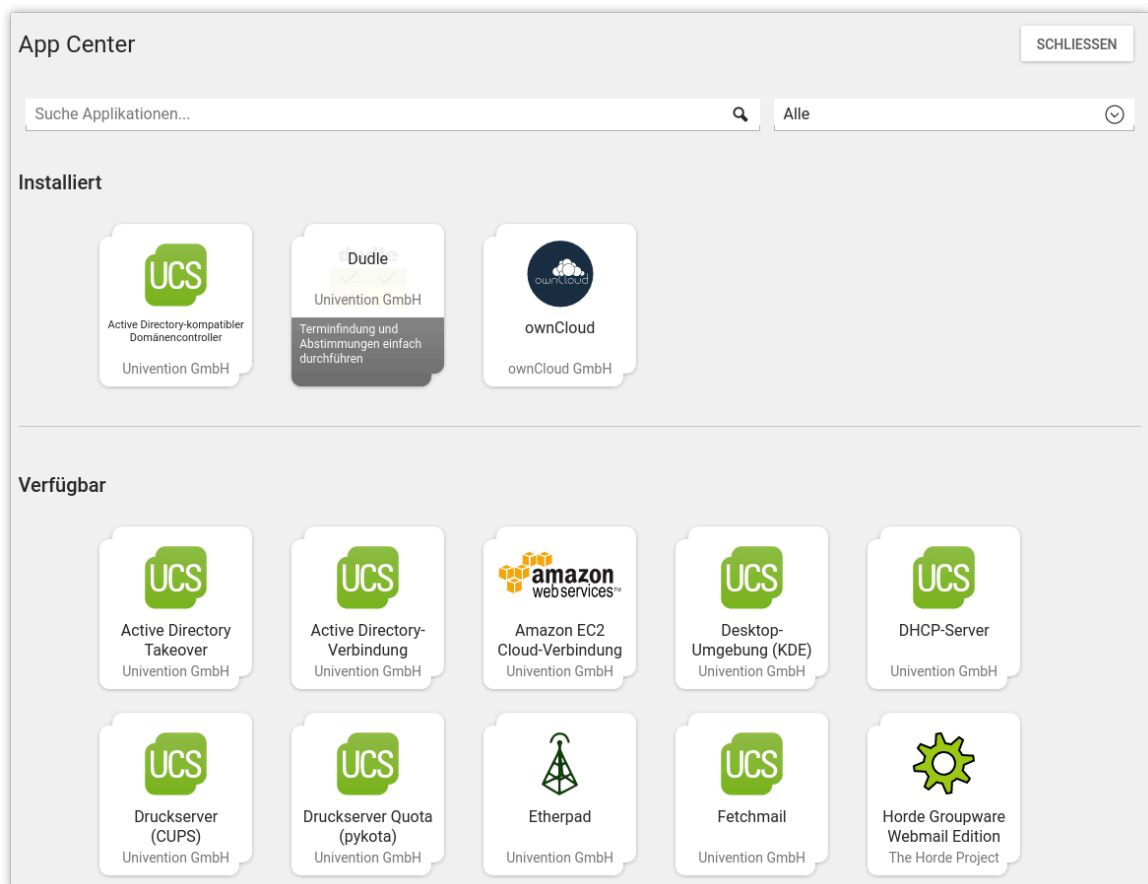
Abbildung 5.1. Überblick der verfügbaren Applikationen im App Center
