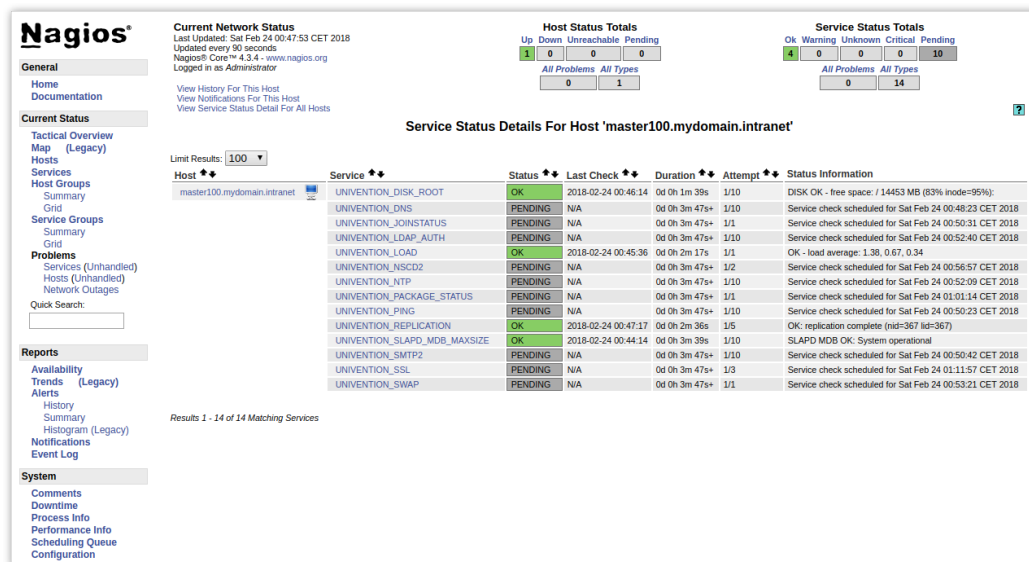
Abbildung 15.3. Nagios Status-Webinterface
