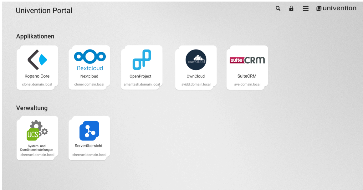
Abbildung 4.1. UCS Portalseite
