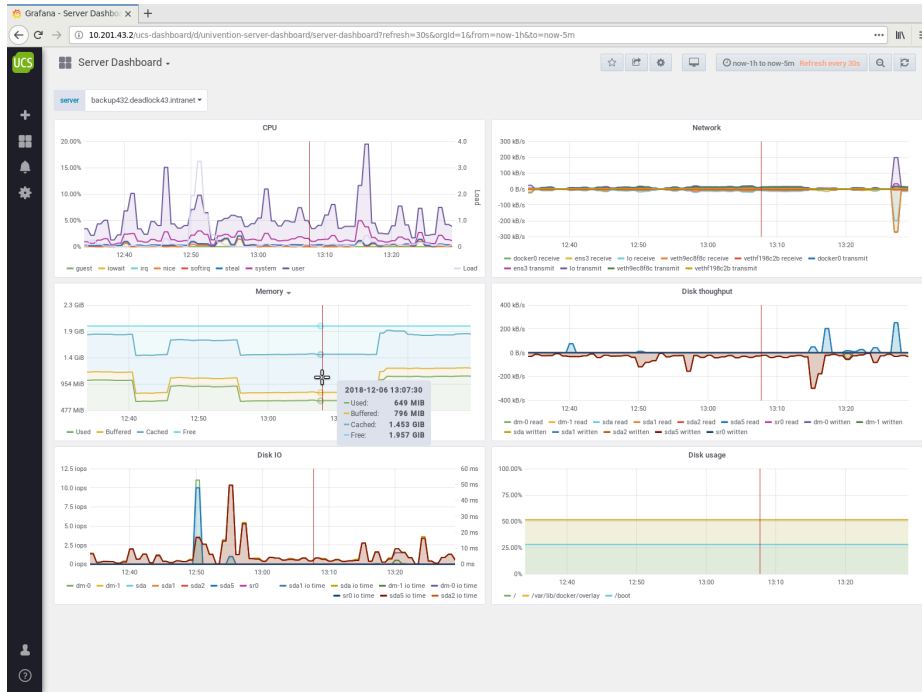
Abbildung 15.2. Server Dashboard
