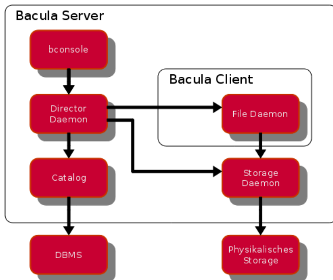
Abbildung 17.1. Bacula Schema
