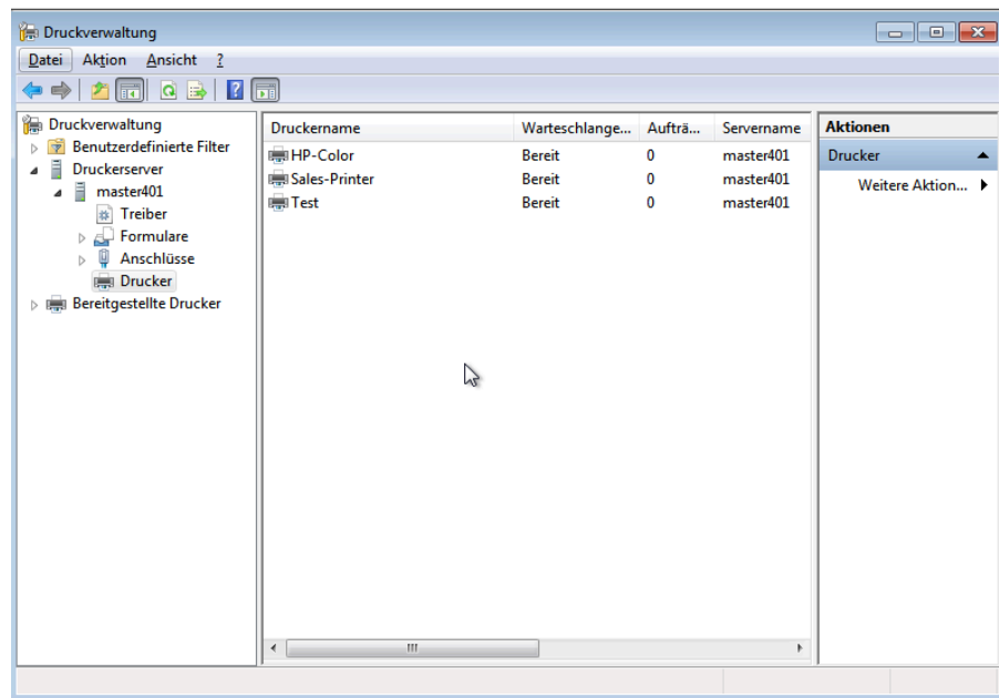
Abbildung 13.5. Druckerliste
