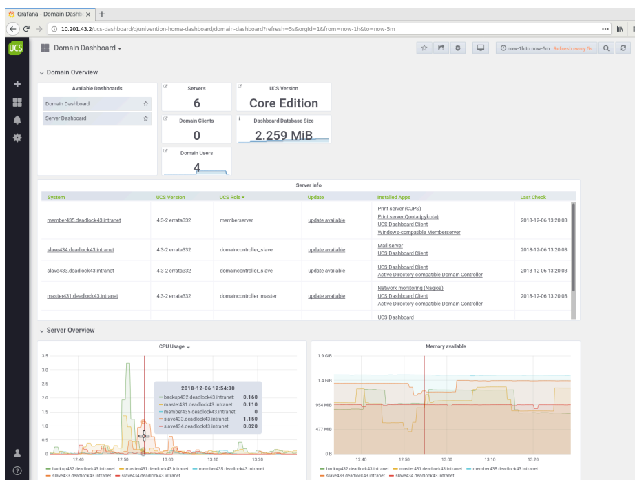
Abbildung 15.1. Domain Dashboard
