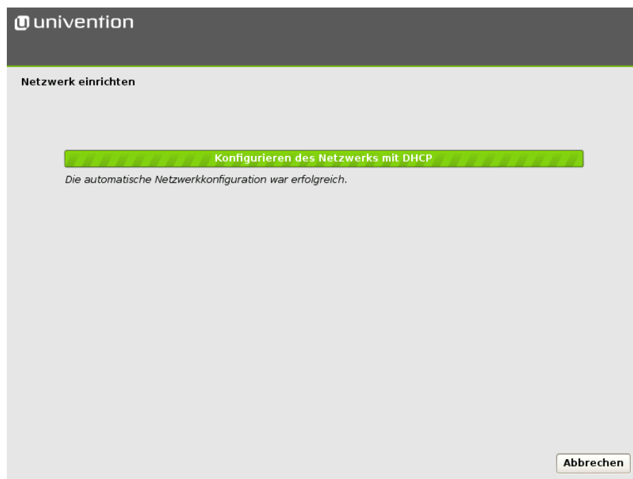
Abbildung 2.5. Automatische Netzwerkkonfiguration
