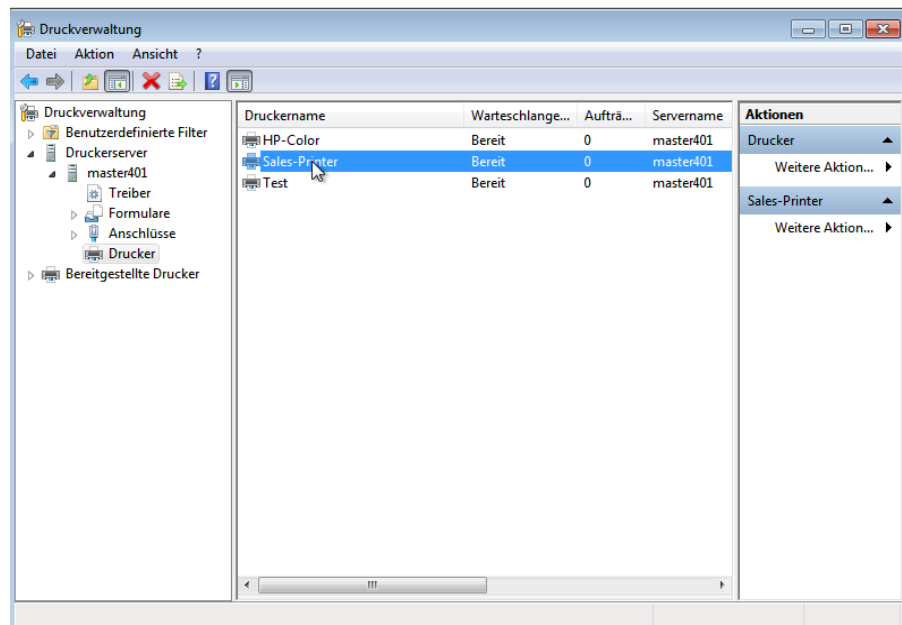
Abbildung 13.7. Drucker auswählen
