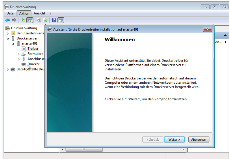
Abbildung 13.6. Treiberinstallation
