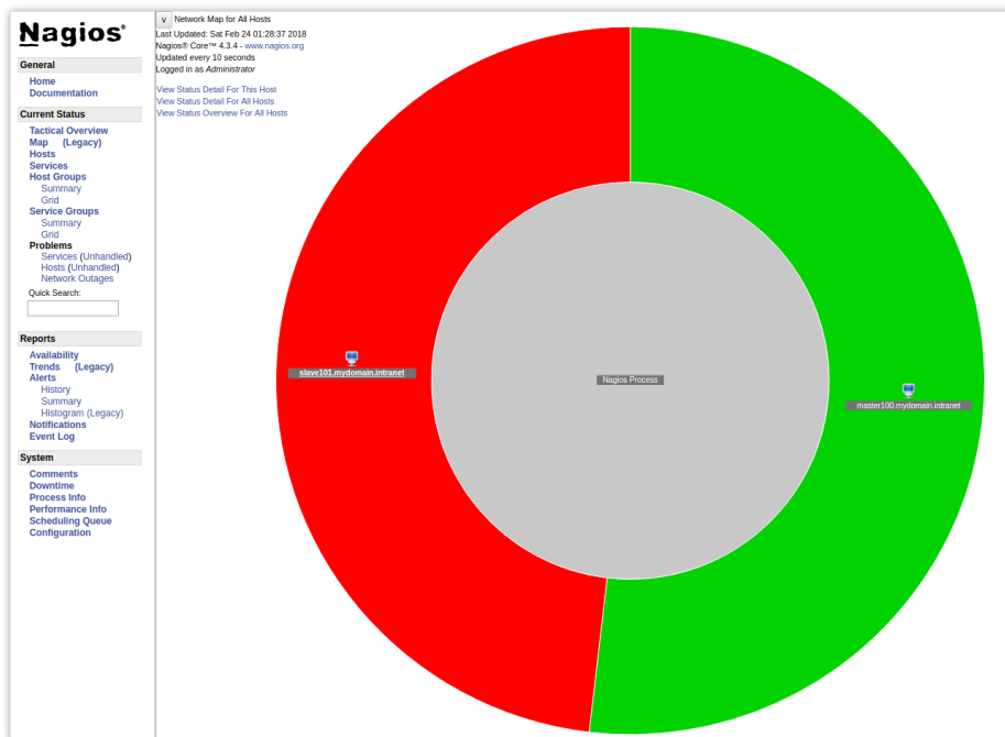
Abbildung 15.6. Nagios-Statusübersicht
