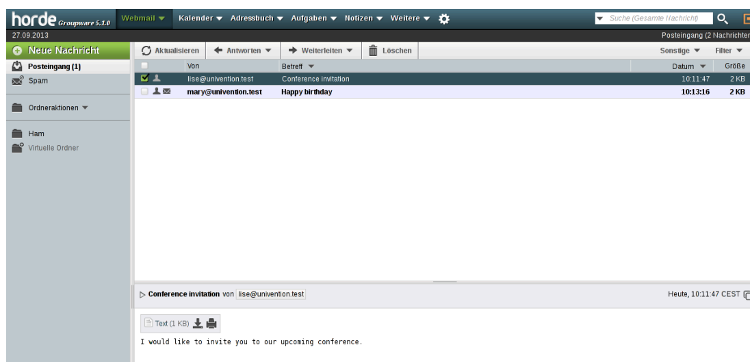
Abbildung 14.5. Webmail (Posteingang)
