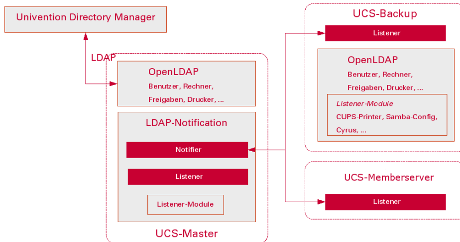
Abbildung 3.3. Listener/Notifier-Mechanismus
