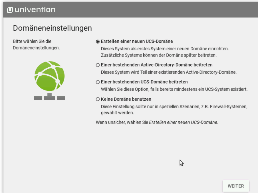
Abbildung 2.11. Domäneneinstellungen
