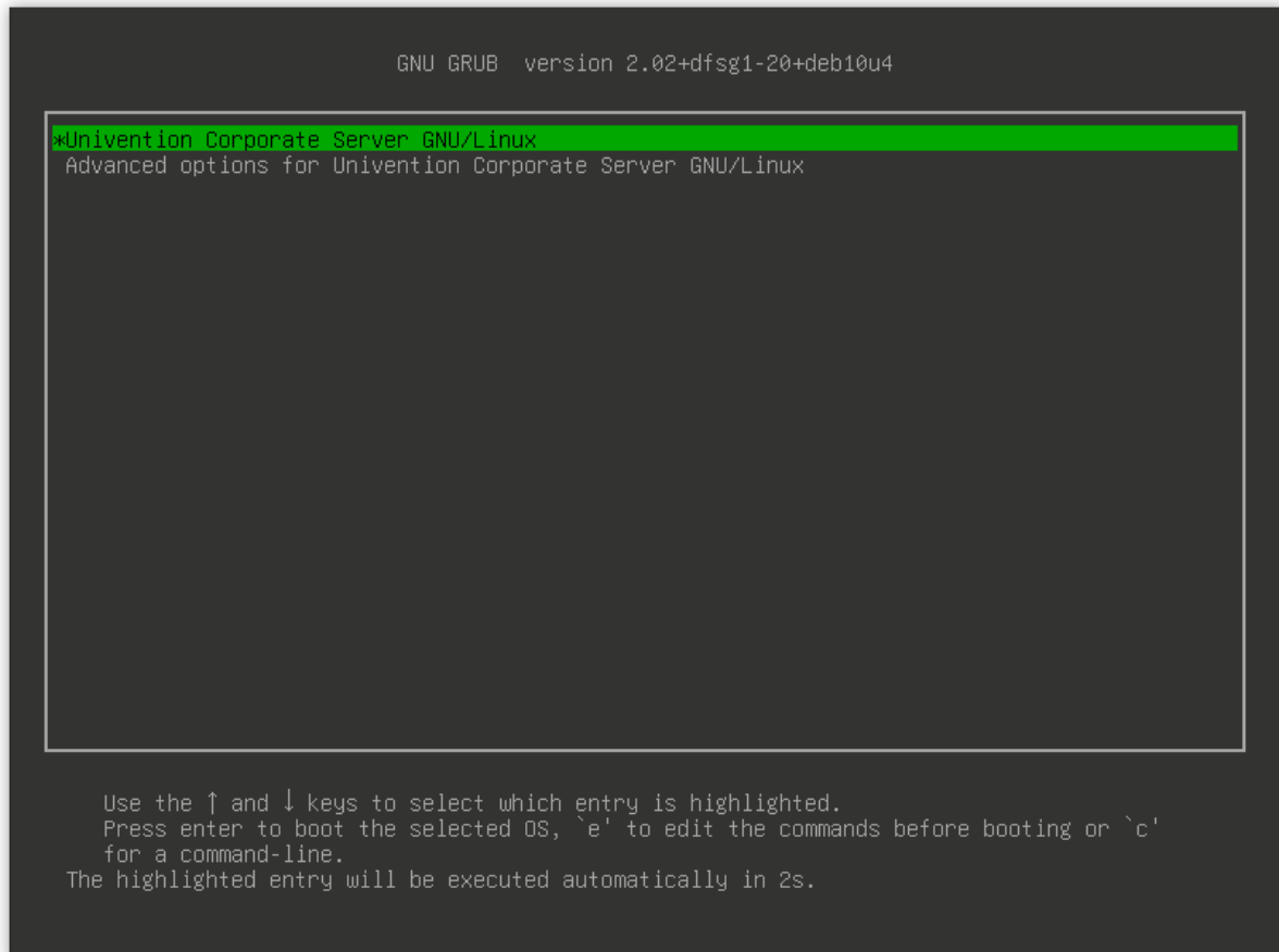
Fig. 8.3: GRUB menu
