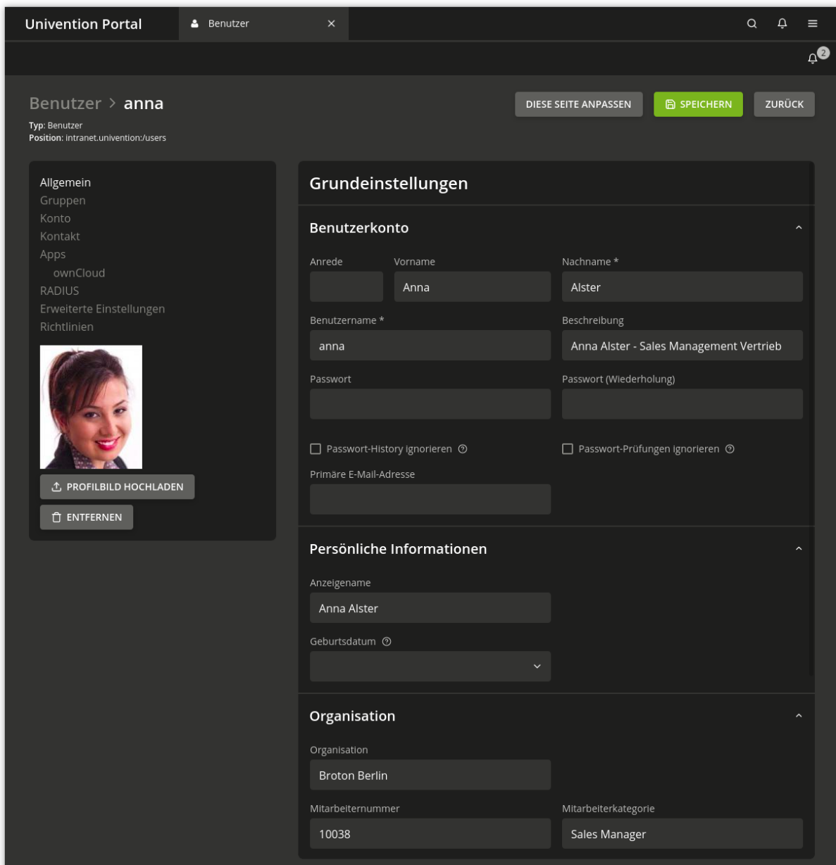
Abb. 6.4: Erweiterte Benutzeransicht
