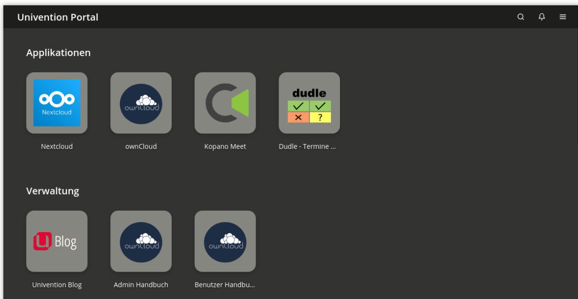
Abb. 4.1: UCS Portalseite
