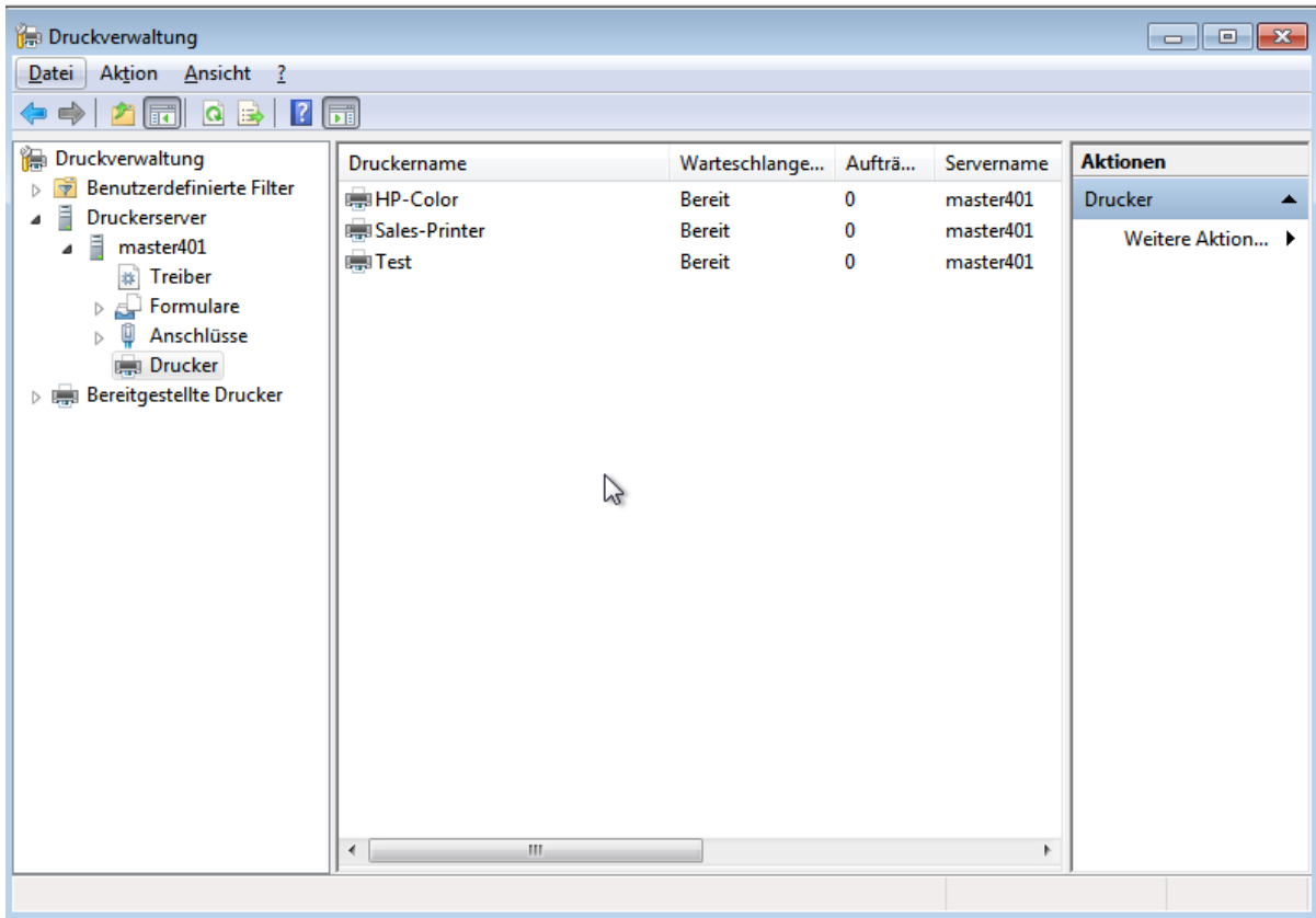
Abb. 13.4: Druckerliste
