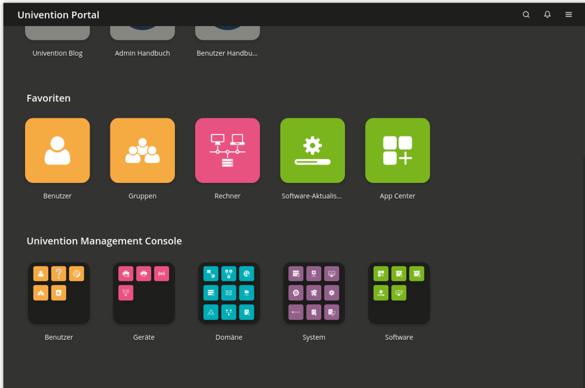
Abb. 4.6: Modulübersicht
