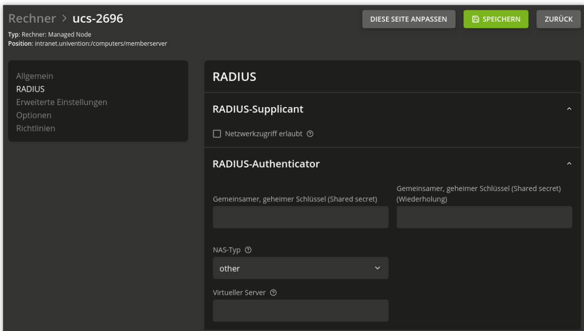
Abb. 11.7: RADIUS-Authenticator Optionen
