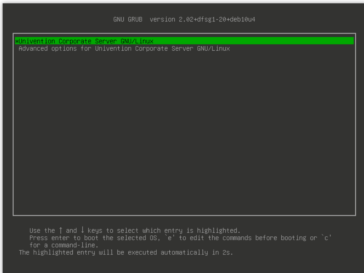
Abb. 8.3: GRUB-Auswahlmenü
