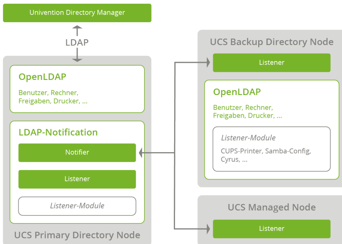
Abb. 3.2: Listener/Notifier-Mechanismus
