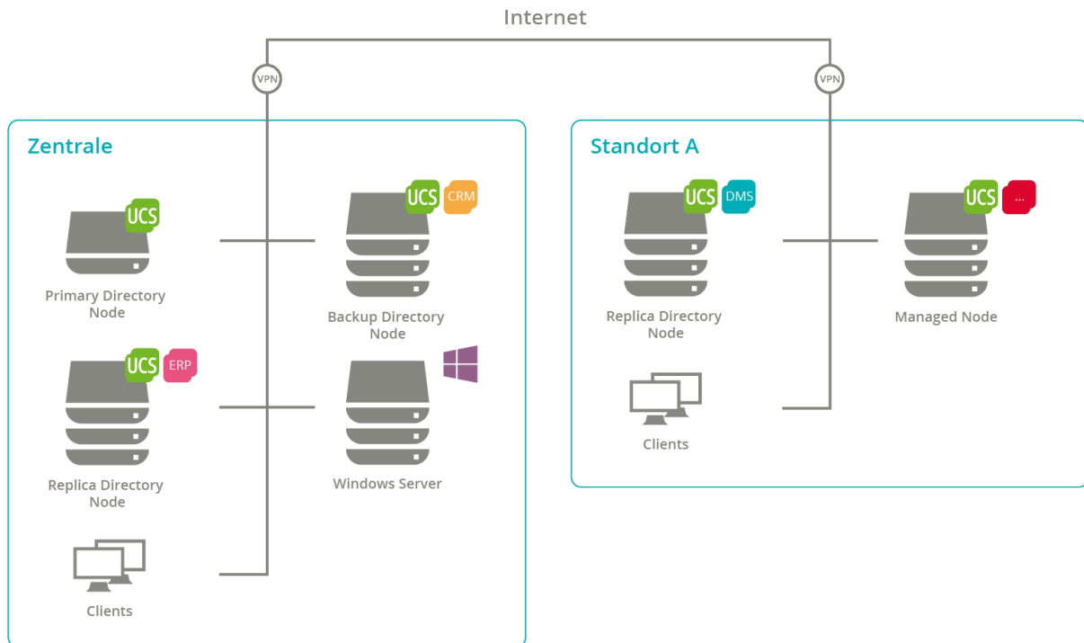
Abb. 1.1: UCS Domänenkonzept
