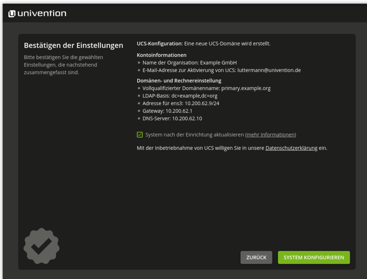
Abb. 2.16: Installationsüberblick
