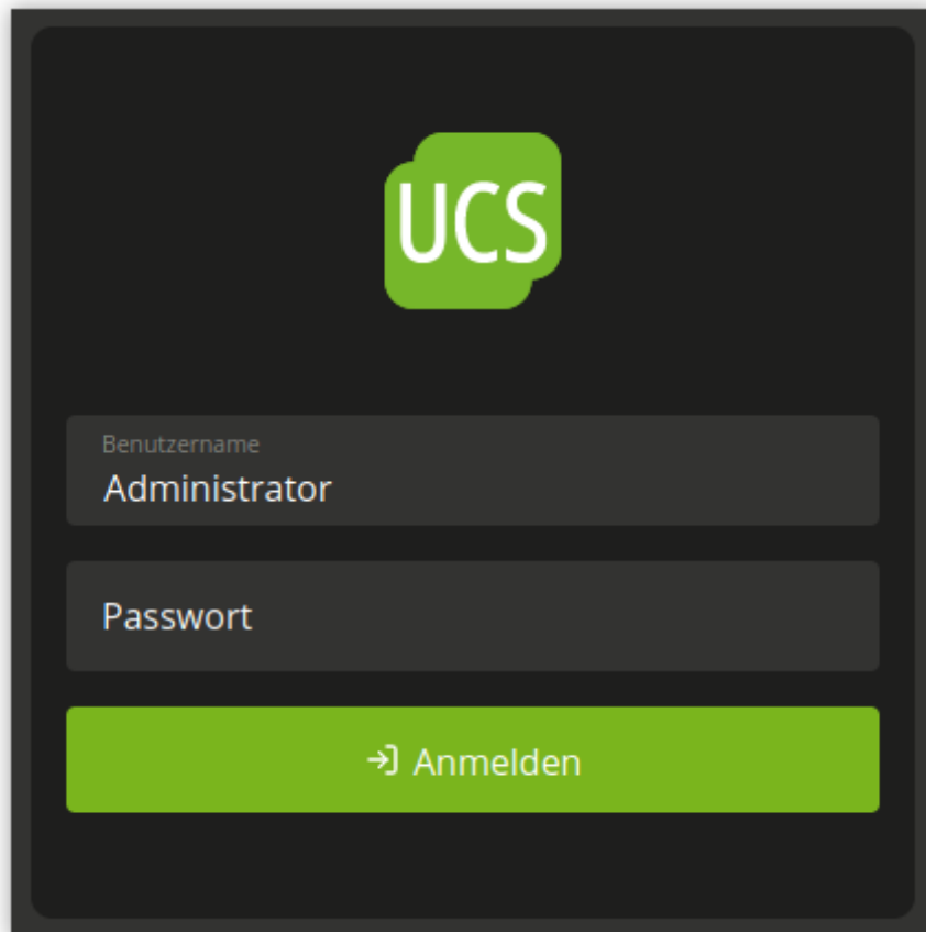
Abb. 4.2: UCS Anmeldeseite
