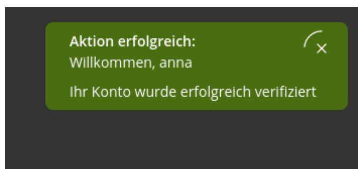
Abb. 6.12: Kontoverifizierung
