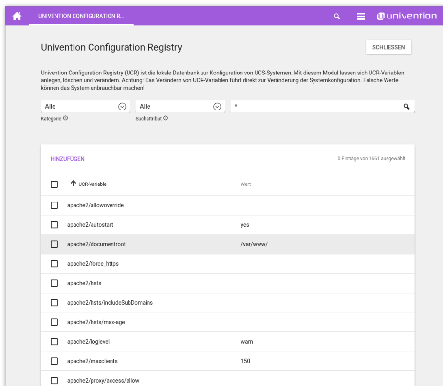
Abbildung 5.1. Verwaltung von Univention Configuration Registry-Variablen
